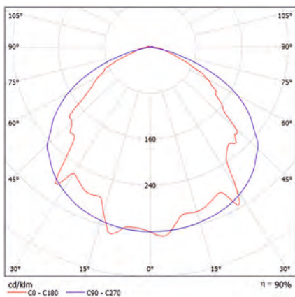
Curva Lumínica
